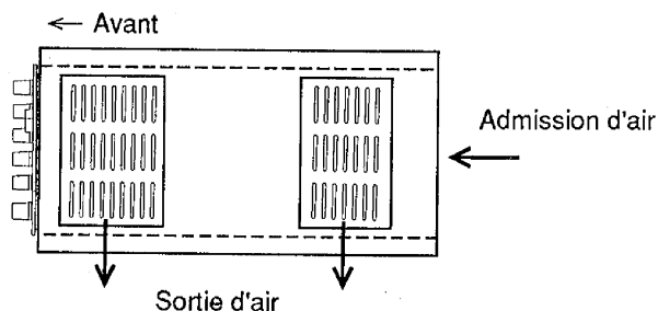
(Vue latérale)
